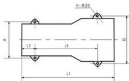
YHCB12-150安装尺寸图 YHCB12-150 mounting dimension drawing
